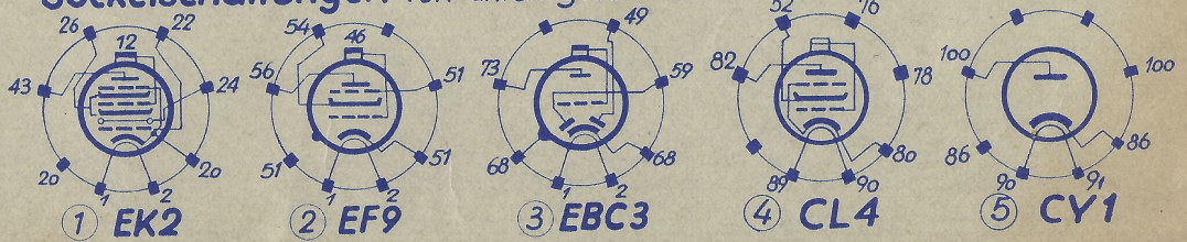
Sockelschaltungen von unten gesehen.
