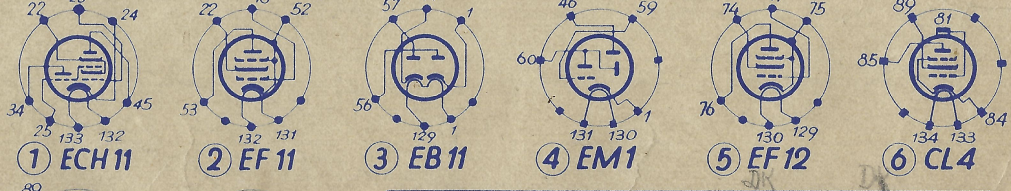
Sockelschaltungen von unten gesehen.
